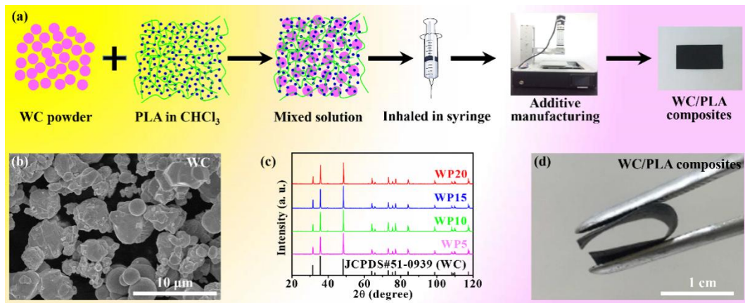
图1 溶液 3D 打印制备碳化钨/聚乳酸复合热电材料示意图(a)；碳化钨的 SEM(b)；碳化钨/聚乳酸复合热电材料的 XRD 谱图(c)；碳化钨/聚乳酸复合热电材料的数码相机照片(d)，其中碳化钨的体积分数为 67%。
