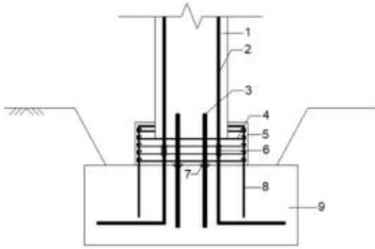
图 2 强震后快速施工桥墩
