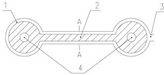
图 4 哑铃形套筒
