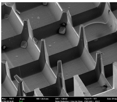
(图1 金属Ni微针SEM图)
